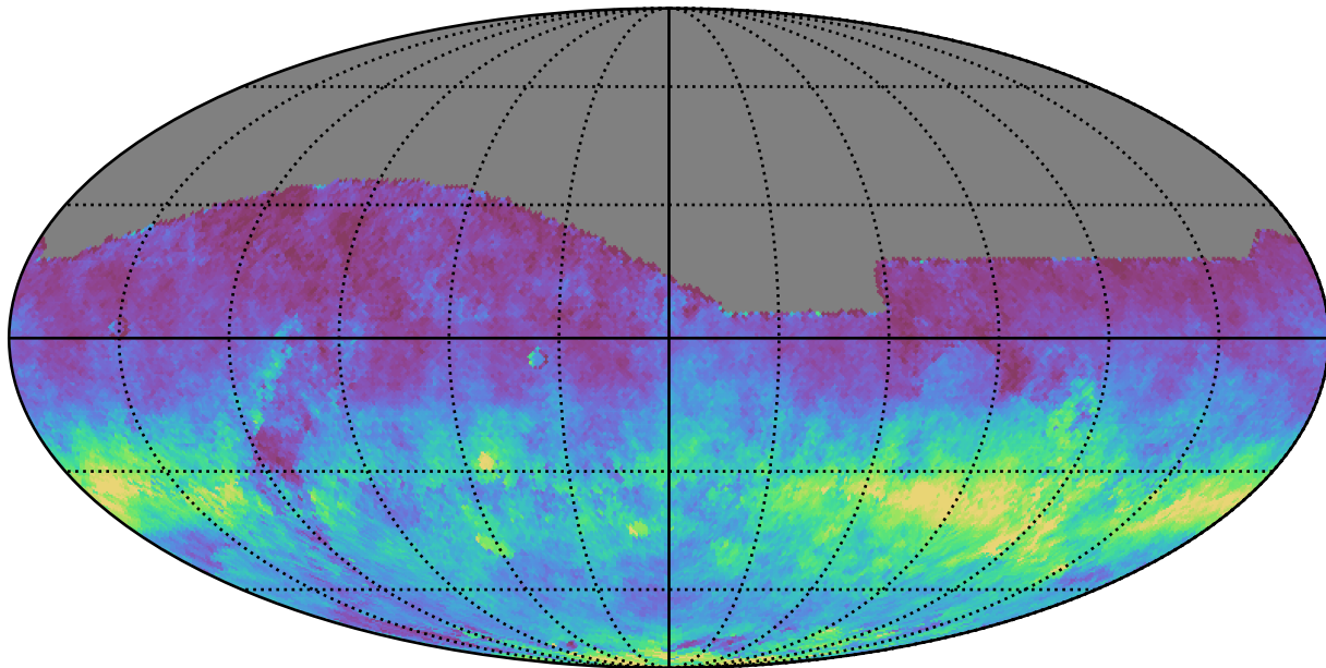
weather_cloudso0v3.4_10yrs All sky i band: AngleRms rotSkyPos
