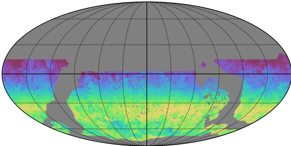
weather_cloudso0v3.4_10yrs WFD z band: AngleRange rotSkyPos
