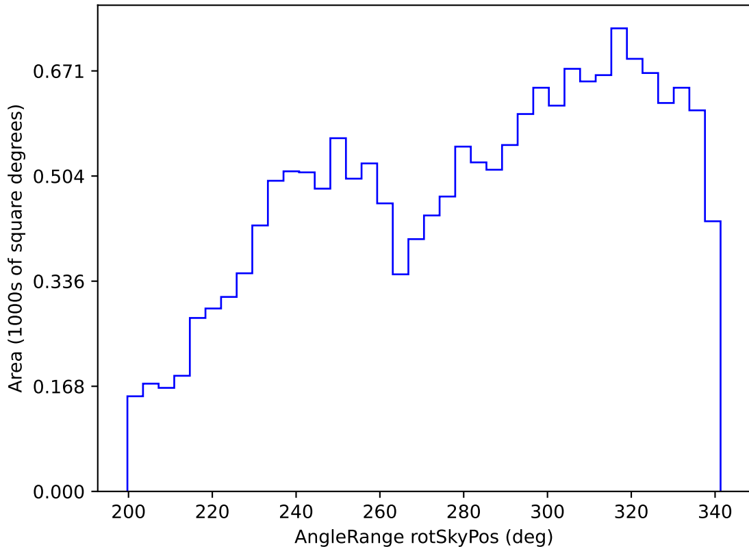
weather_cloudso0v3.4_10yrs WFD z band: AngleRange rotSkyPos
