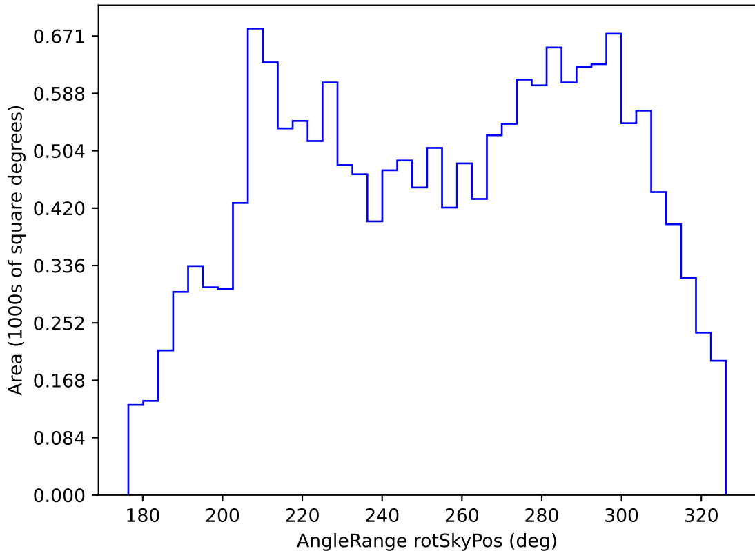
weather_cloudso0v3.4_10yrs WFD u band: AngleRange rotSkyPos
