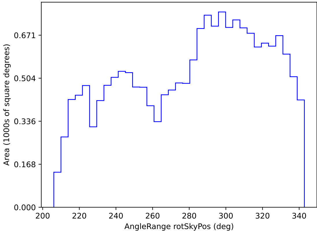
weather_cloudso0v3.4_10yrs WFD r band: AngleRange rotSkyPos
