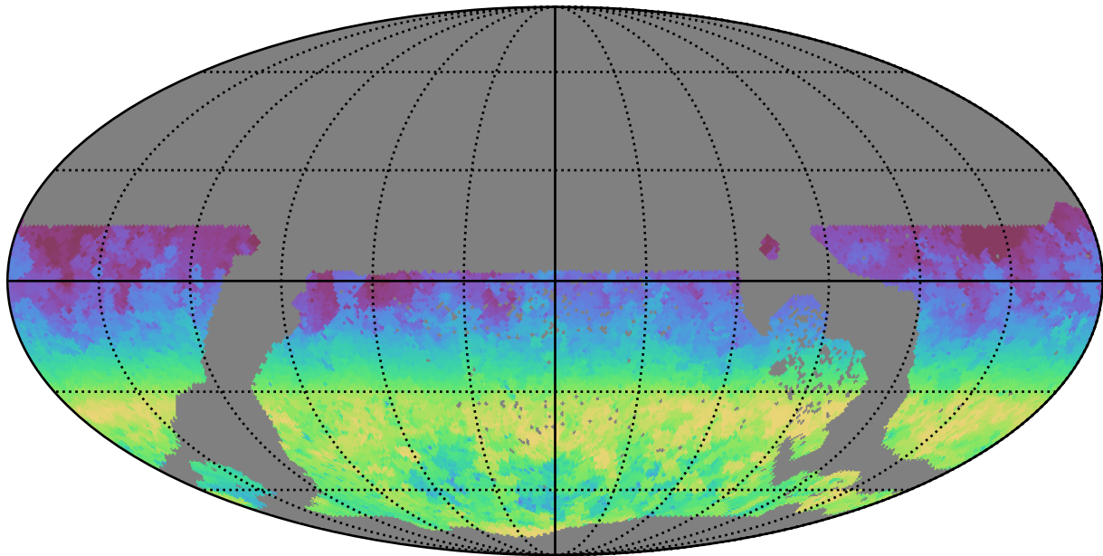
weather_cloudso0v3.4_10yrs WFD i band: AngleRange rotSkyPos
