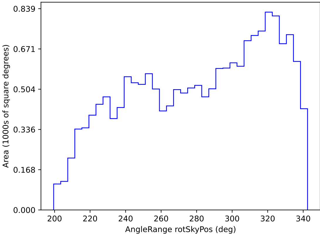
weather_cloudso0v3.4_10yrs WFD i band: AngleRange rotSkyPos
