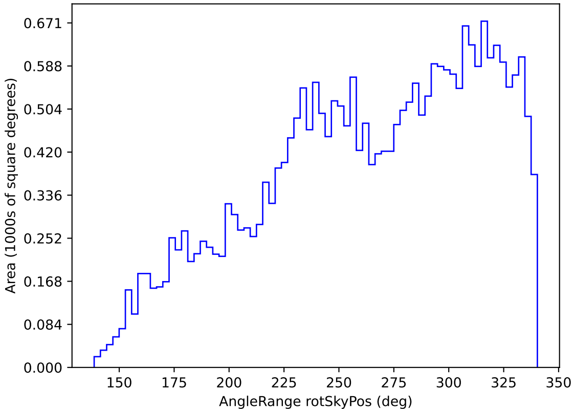
weather_cloudso0v3.4_10yrs All sky z band: AngleRange rotSkyPos
