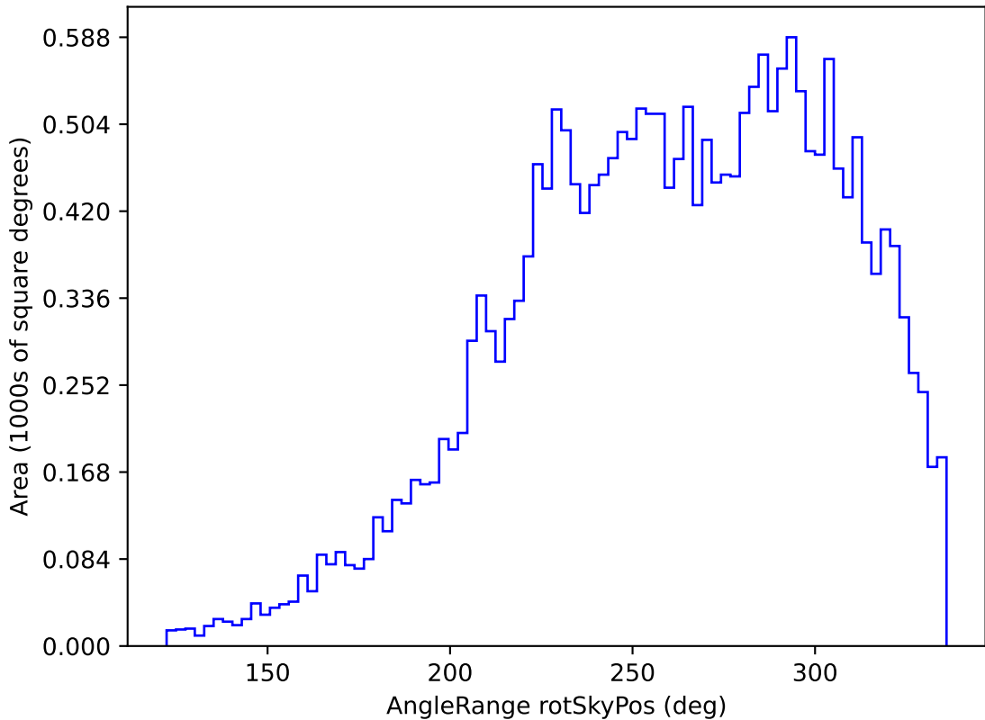
weather_cloudso0v3.4_10yrs All sky y band: AngleRange rotSkyPos
