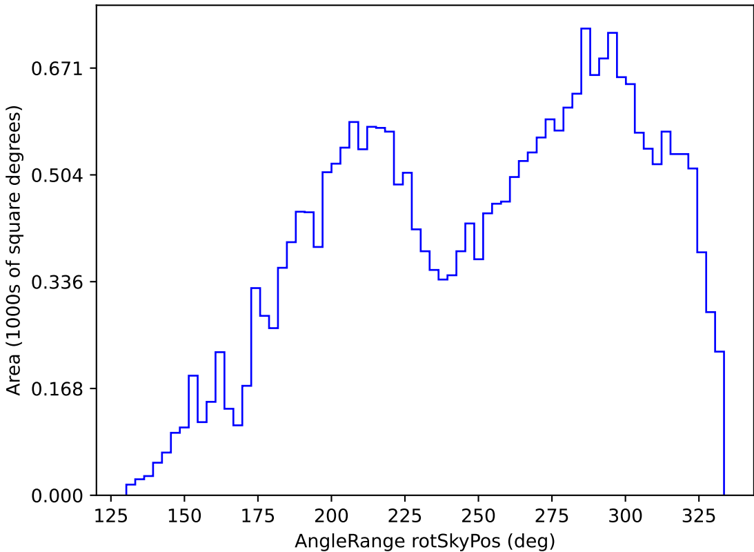
weather_cloudso0v3.4_10yrs All sky g band: AngleRange rotSkyPos
