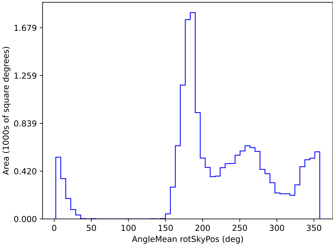
weather_cloudso0v3.4_10yrs WFD y band: AngleMean rotSkyPos
