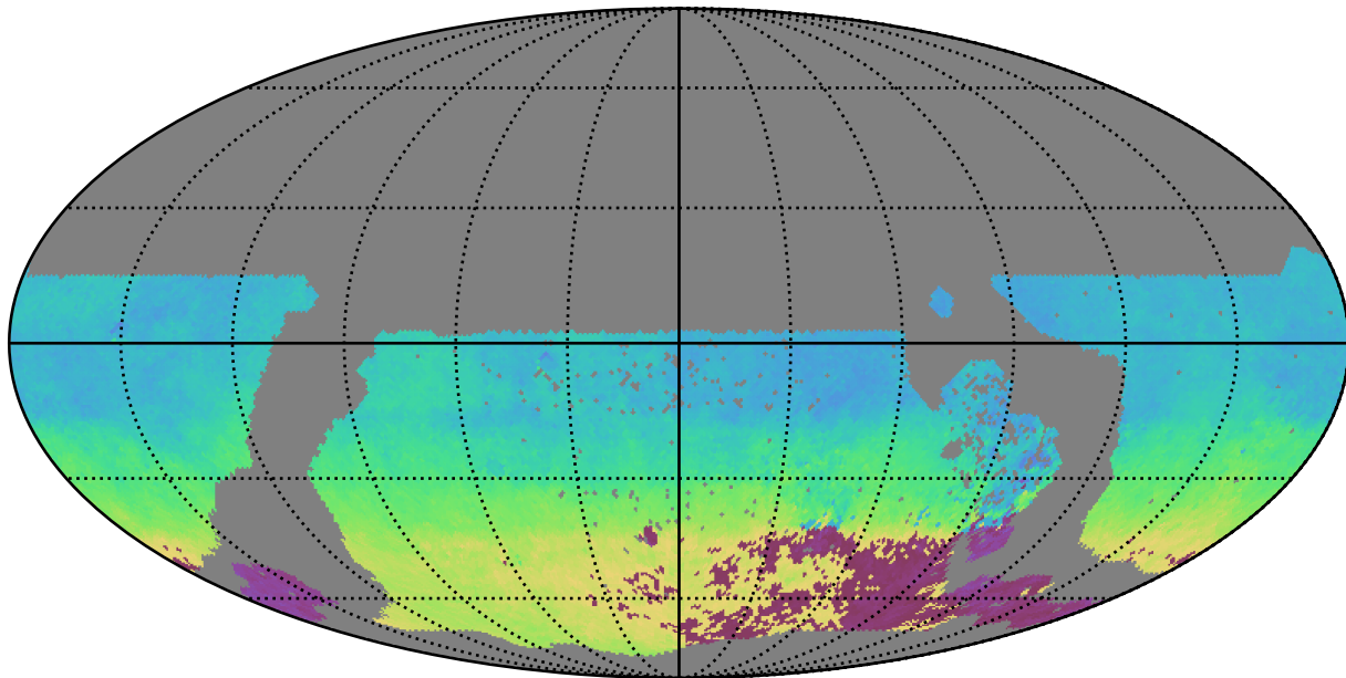
weather_cloudso0v3.4_10yrs WFD u band: AngleMean rotSkyPos
