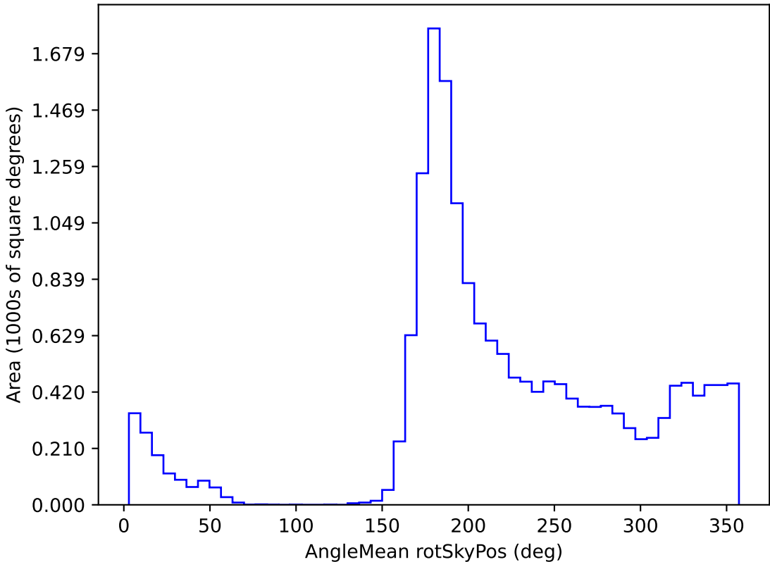
weather_cloudso0v3.4_10yrs WFD u band: AngleMean rotSkyPos
