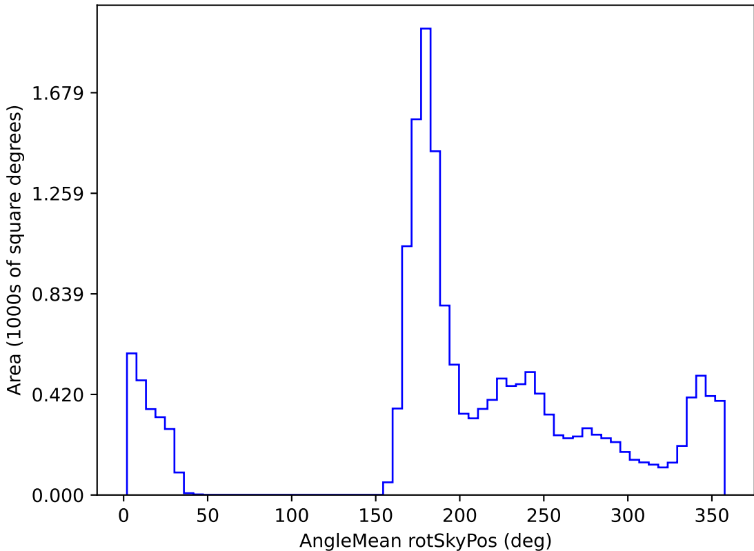
weather_cloudso0v3.4_10yrs WFD r band: AngleMean rotSkyPos
