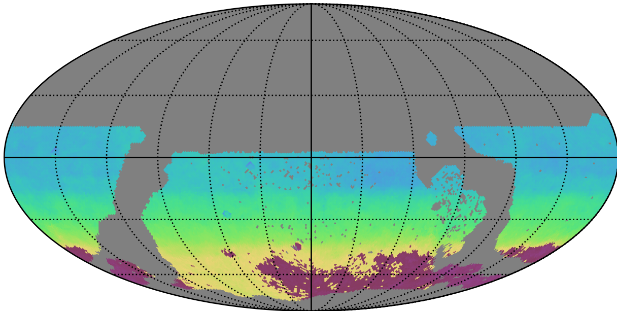
weather_cloudso0v3.4_10yrs WFD i band: AngleMean rotSkyPos
