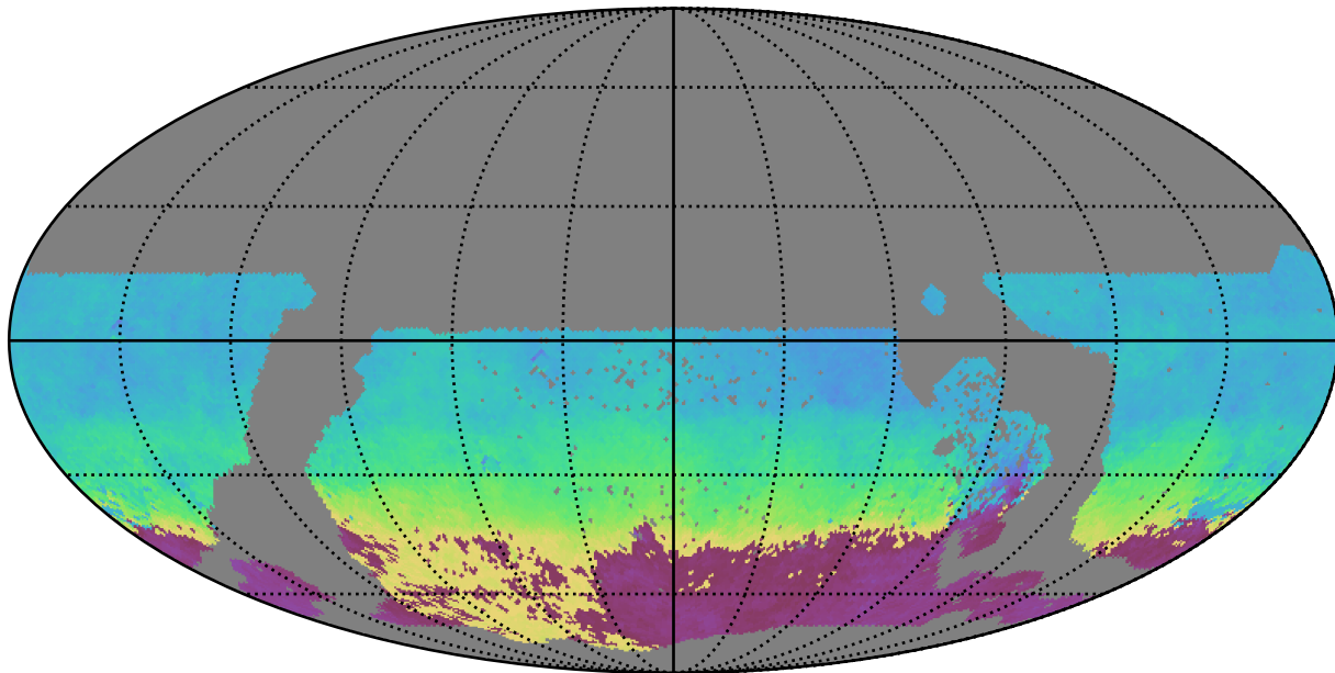
weather_cloudso0v3.4_10yrs WFD g band: AngleMean rotSkyPos
