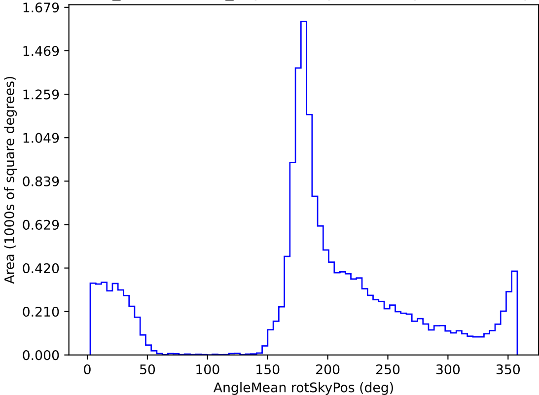
weather_cloudso0v3.4_10yrs WFD g band: AngleMean rotSkyPos
