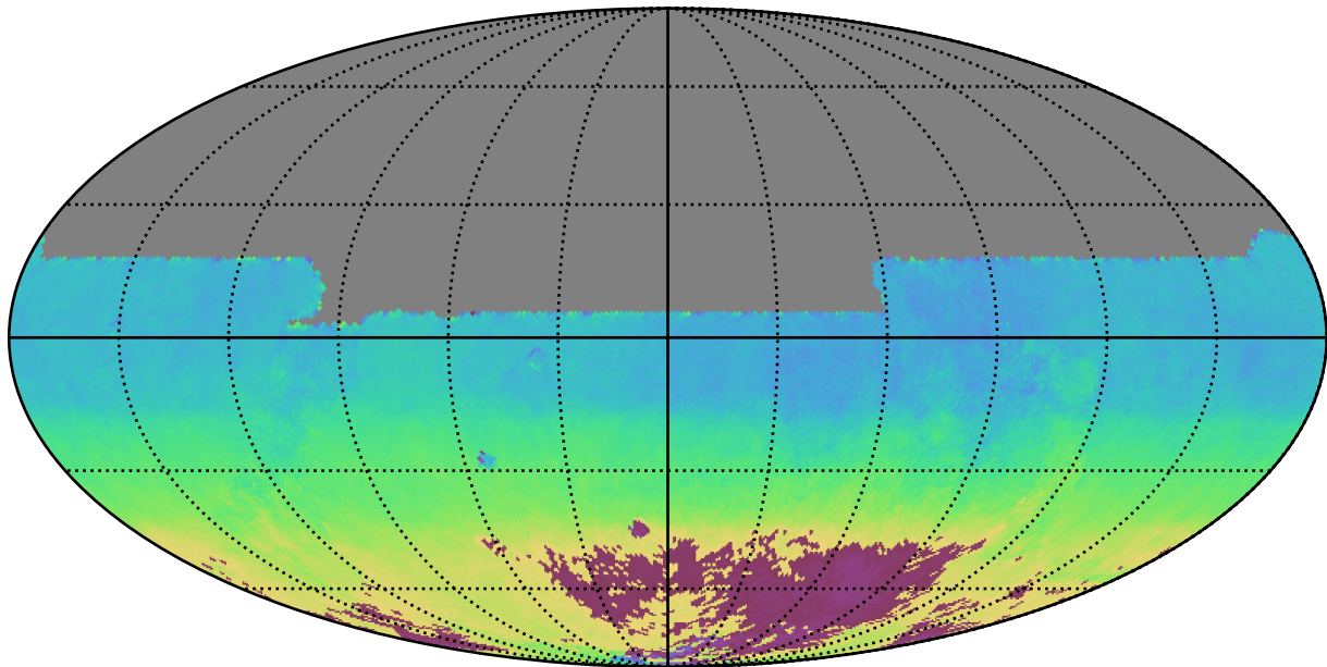
weather_cloudso0v3.4_10yrs All sky y band: AngleMean rotSkyPos
