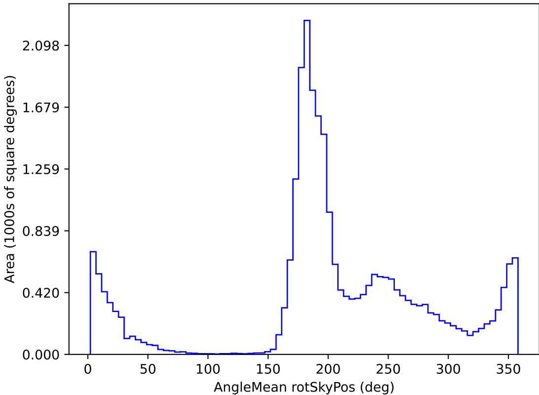
weather_cloudso0v3.4_10yrs All sky i band: AngleMean rotSkyPos
