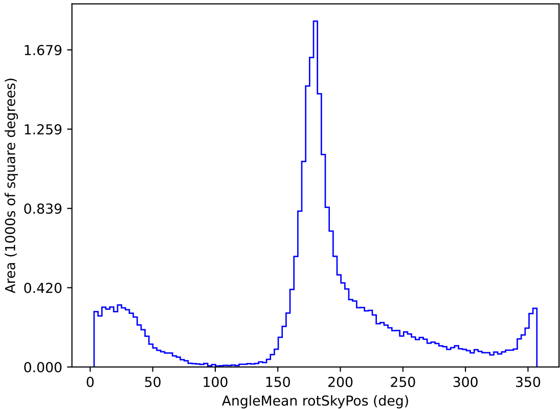
weather_cloudso0v3.4_10yrs All sky g band: AngleMean rotSkyPos
