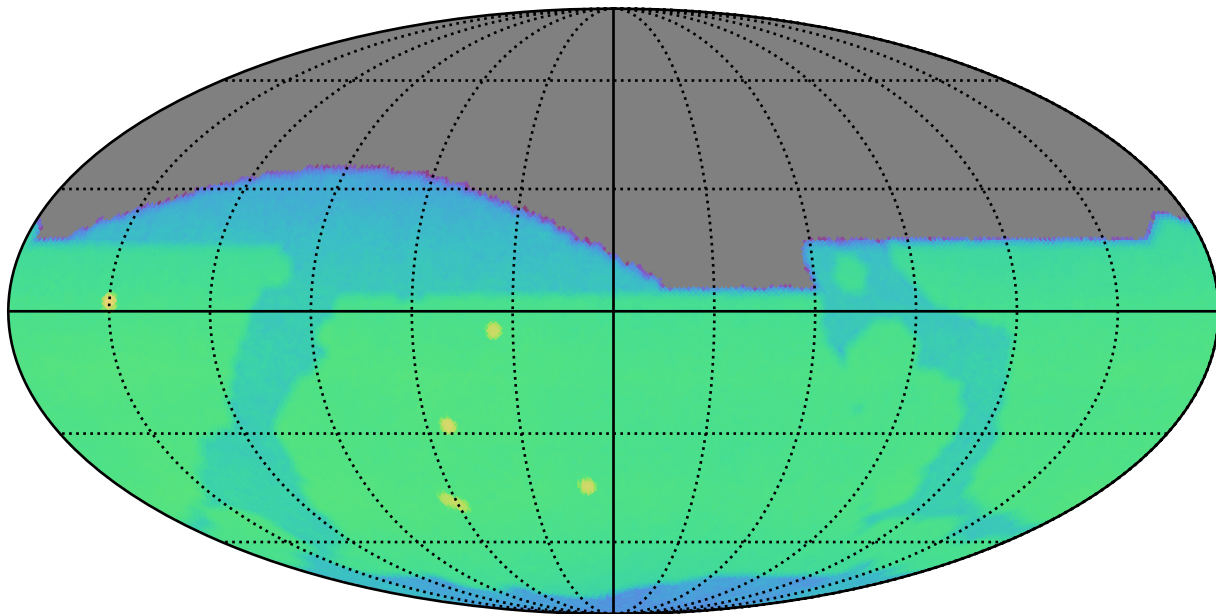
weather_cloudso0v3.4_10yrs i: CoaddM5
