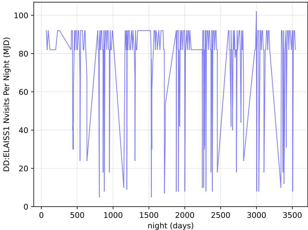
weather_cloudso0v3.4_10yrs all bands: DD:ELAISS1 Nvisits Per Night
