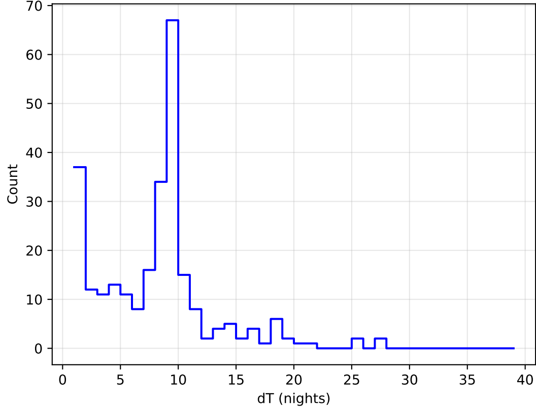
weather_cloudso0v3.4_10yrs all bands: DD:ELAISS1 Delta Nights Histogram
