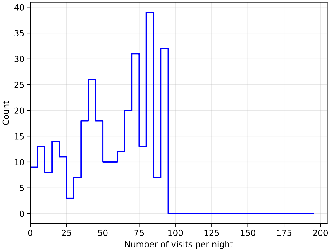
weather_cloudso0v3.4_10yrs all bands: DD:EDFS NVisitsPerNight
