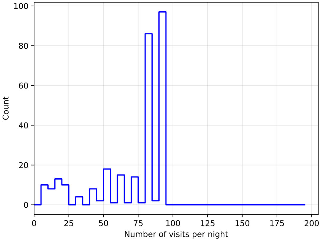
weather_cloudso0v3.4_10yrs all bands: DD:ECDFS NVisitsPerNight
