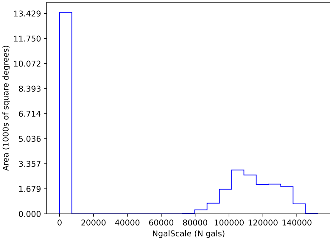
too_ignore_5_4v3.4_10yrs i: NgalScale
