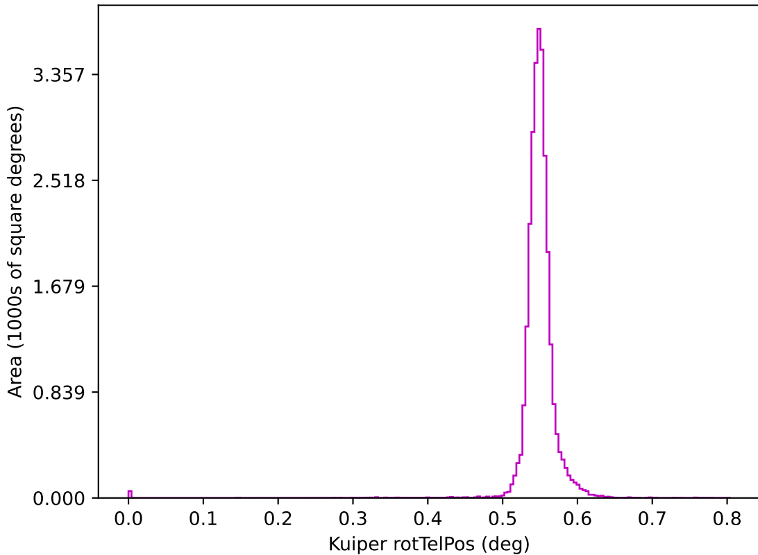
too_ignore_5_4v3.4_10yrs z: Kuiper rotTelPos
