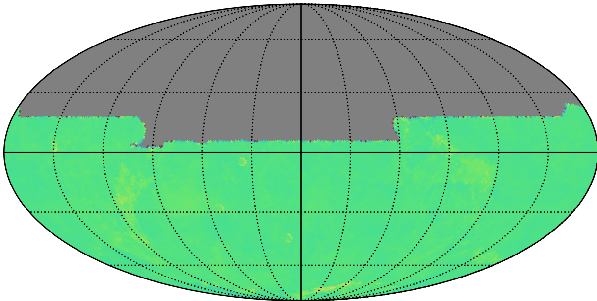
too_ignore_5_4v3.4_10yrs y: Kuiper rotTelPos
