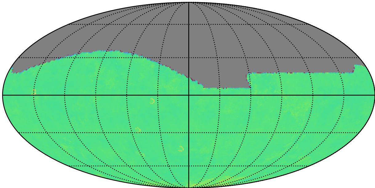
too_ignore_5_4v3.4_10yrs r: Kuiper rotTelPos
