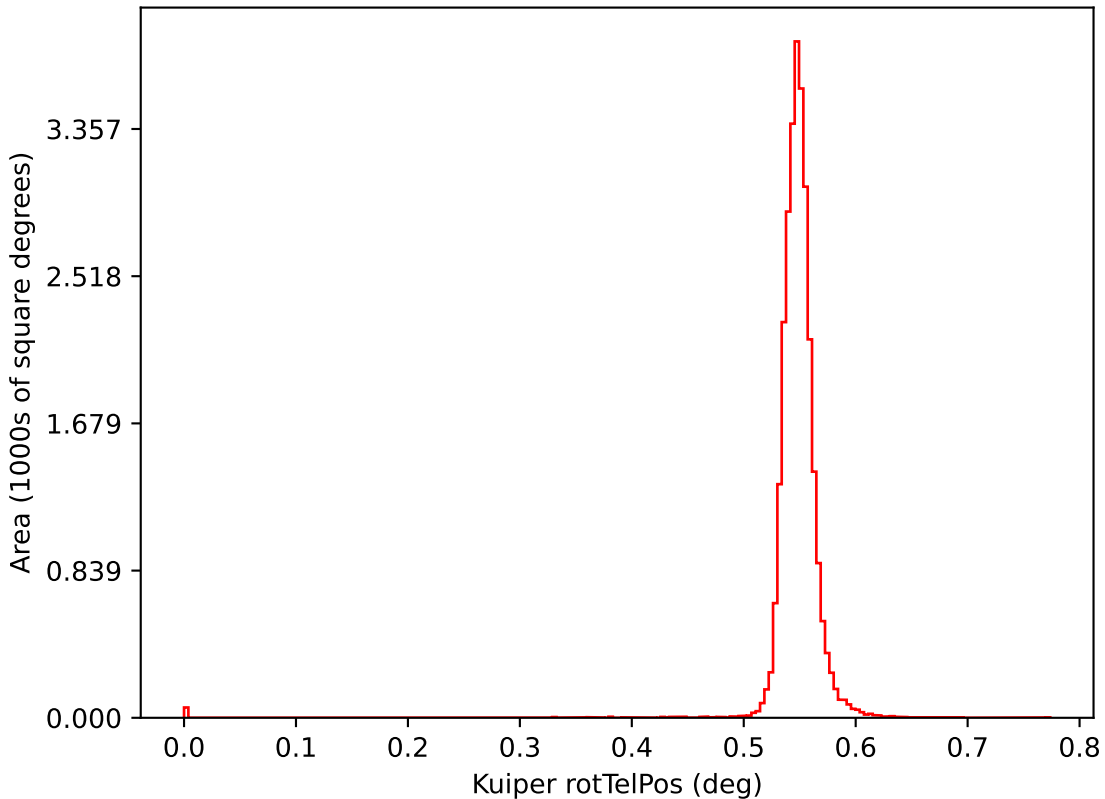
too_ignore_5_4v3.4_10yrs i: Kuiper rotTelPos
