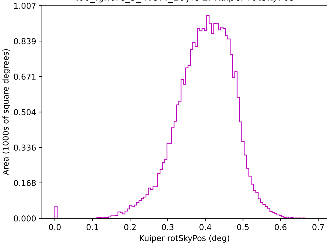
too_ignore_5_4v3.4_10yrs z: Kuiper rotSkyPos
