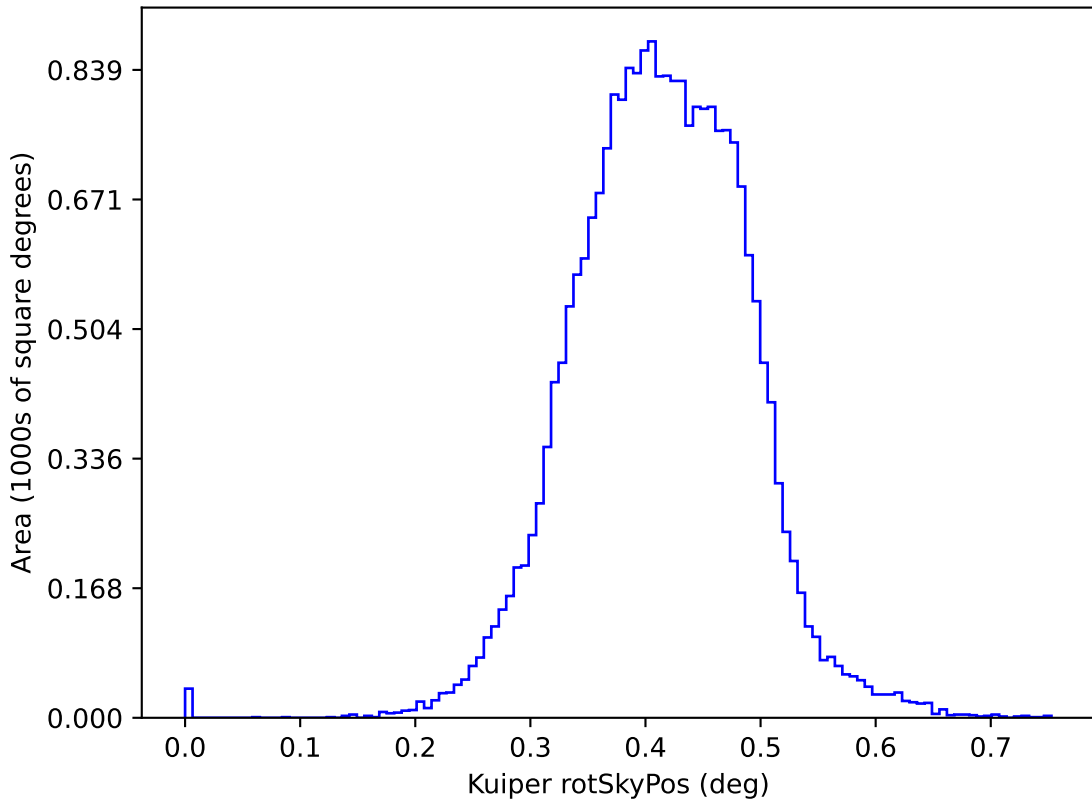
too_ignore_5_4v3.4_10yrs y: Kuiper rotSkyPos
