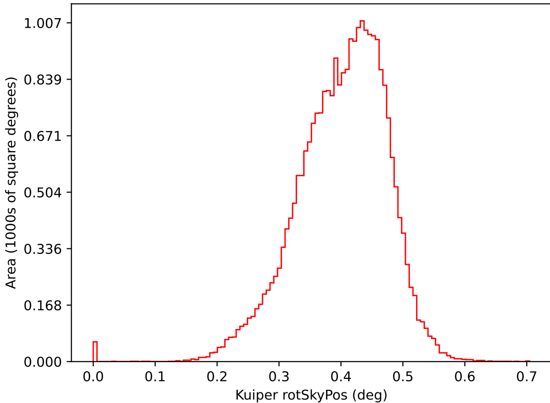
too_ignore_5_4v3.4_10yrs i: Kuiper rotSkyPos
