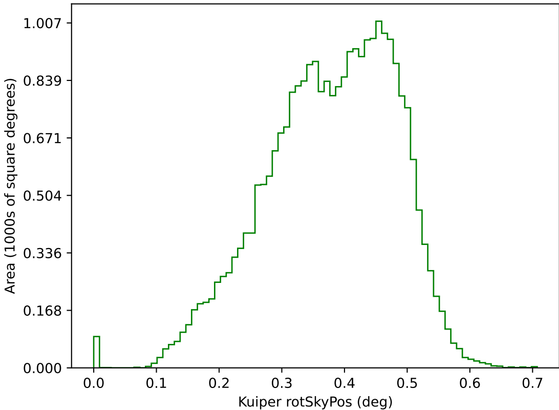
too_ignore_5_4v3.4_10yrs g: Kuiper rotSkyPos
