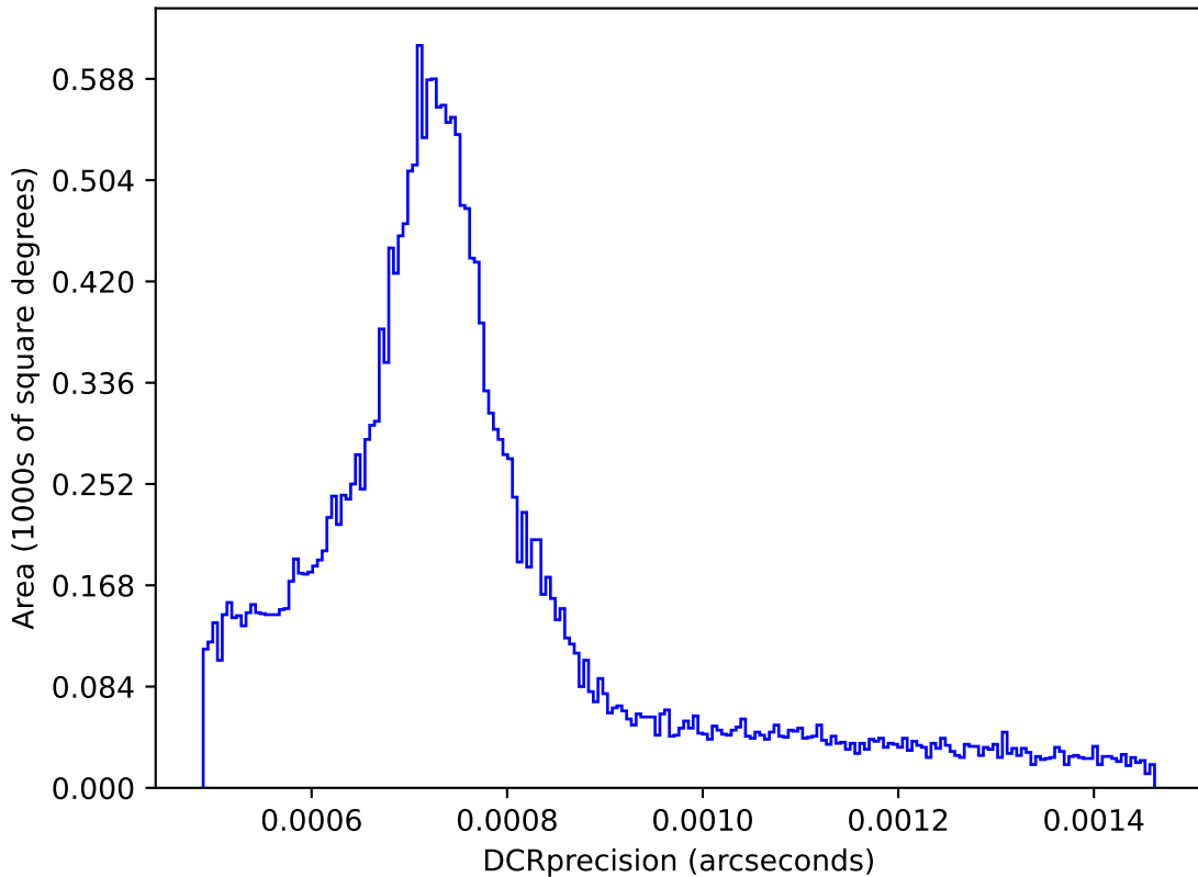
too_ignore_5_4v3.4_10yrs : DCRprecision
