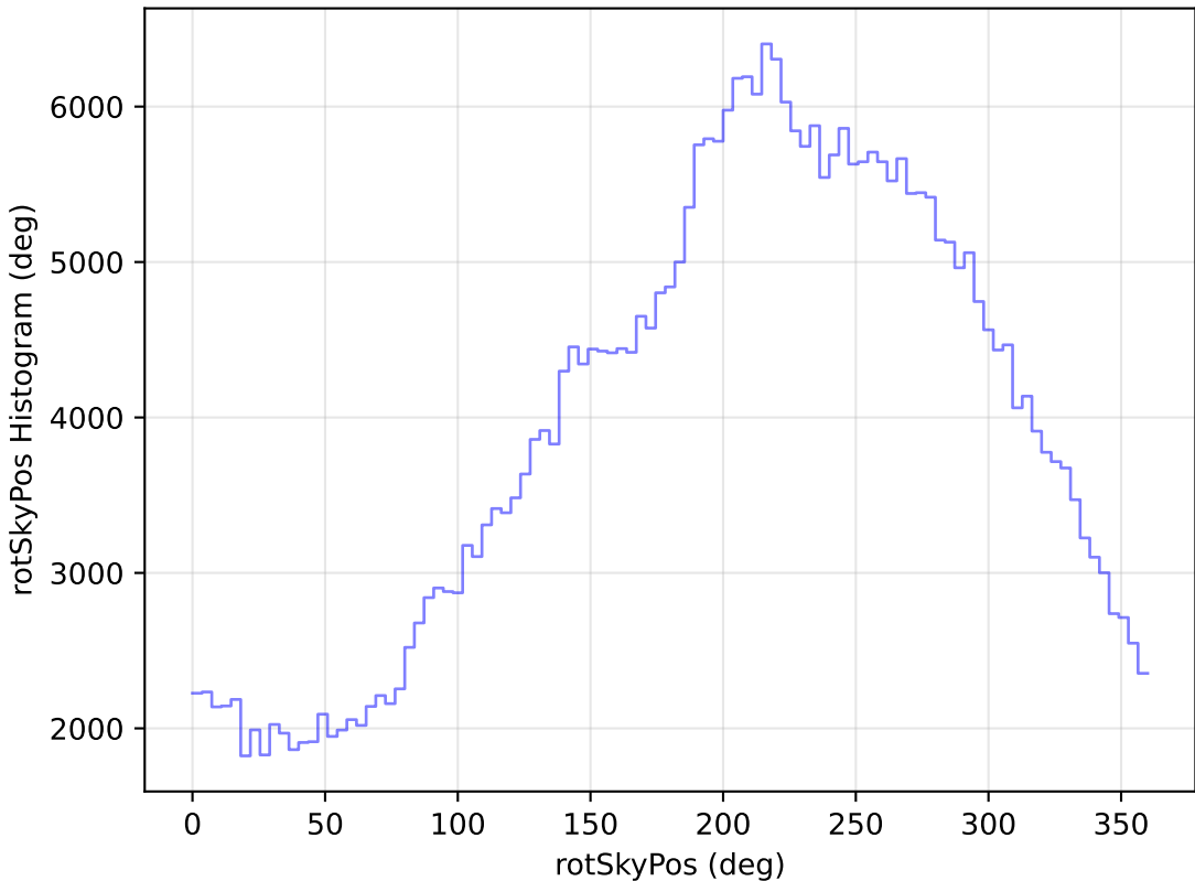
too_ignore_5_4v3.4_10yrs WFD y band: rotSkyPos Histogram
