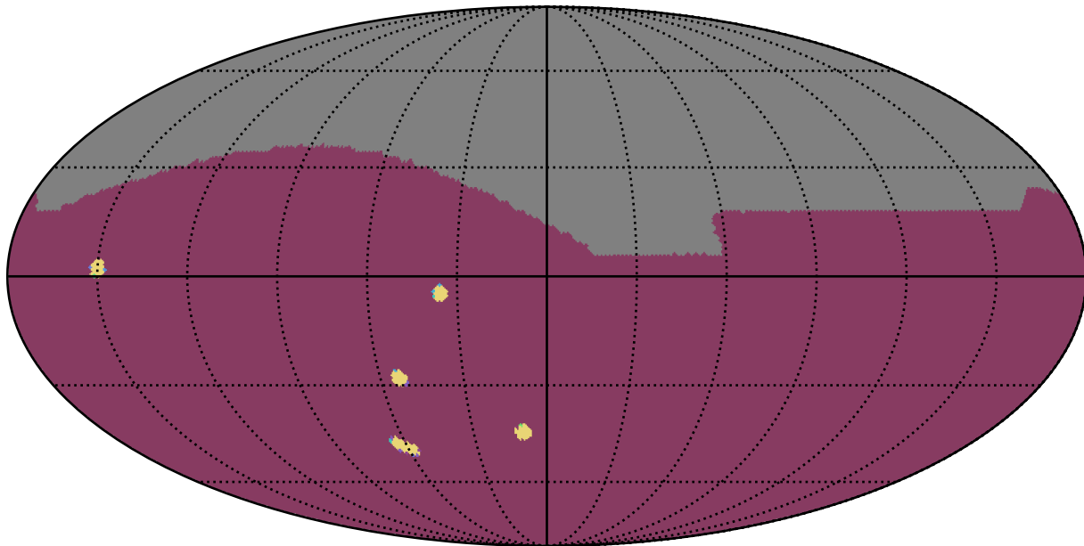
too_ignore_5_4v3.4_10yrs All sky: NumberOfQuickRevisits
