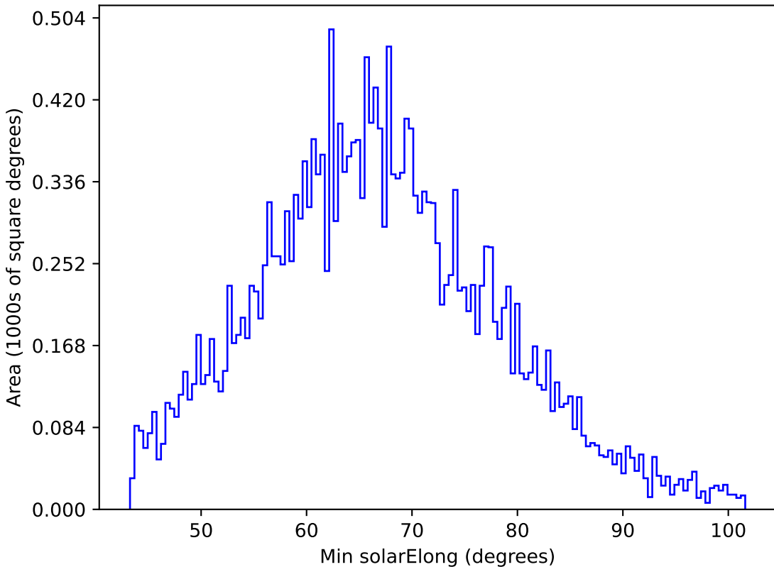
too_ignore_5_4v3.4_10yrs All sky y band: Min solarElong
