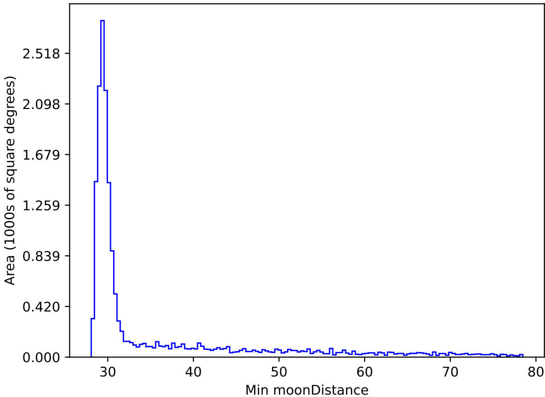
too_ignore_5_4v3.4_10yrs WFD y band: Min moonDistance
