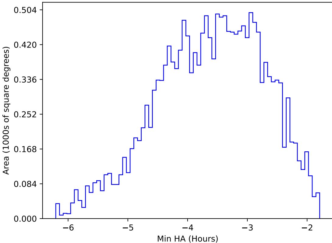
too_ignore_5_4v3.4_10yrs WFD y band: Min HA
