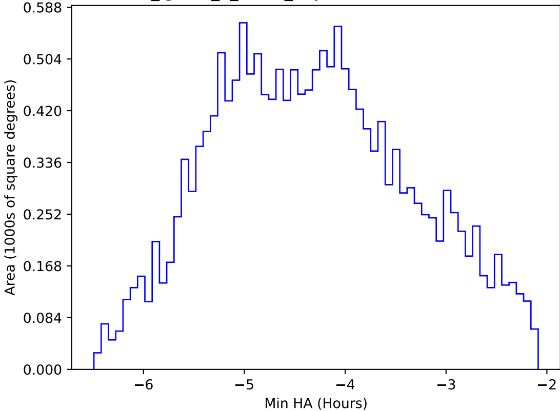
too_ignore_5_4v3.4_10yrs WFD i band: Min HA
