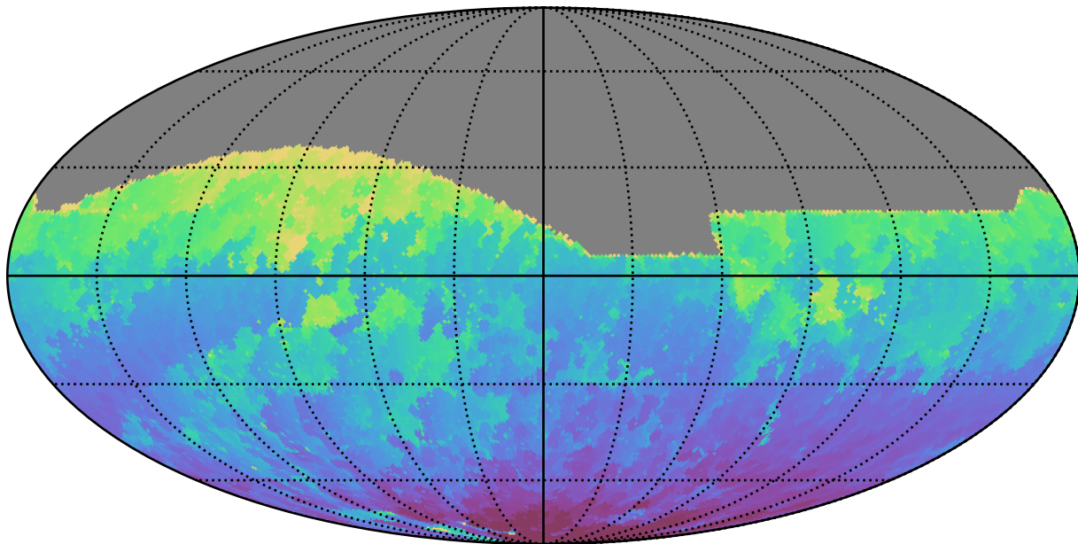
too_ignore_5_4v3.4_10yrs All sky z band: Min HA
