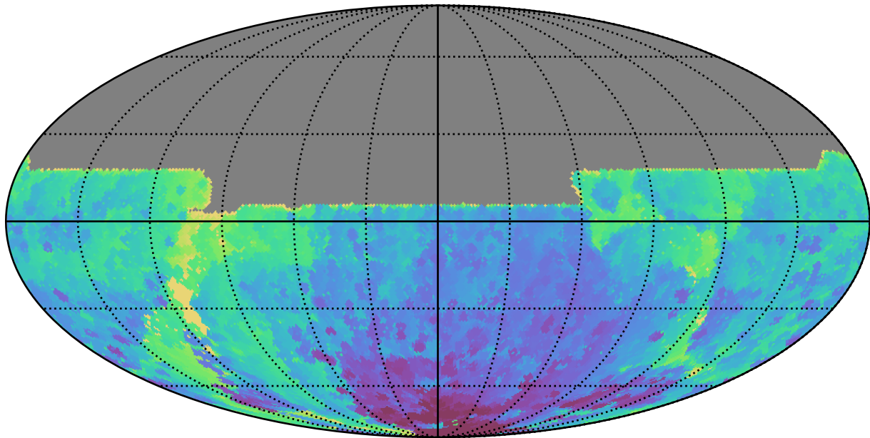
too_ignore_5_4v3.4_10yrs All sky y band: Min HA
