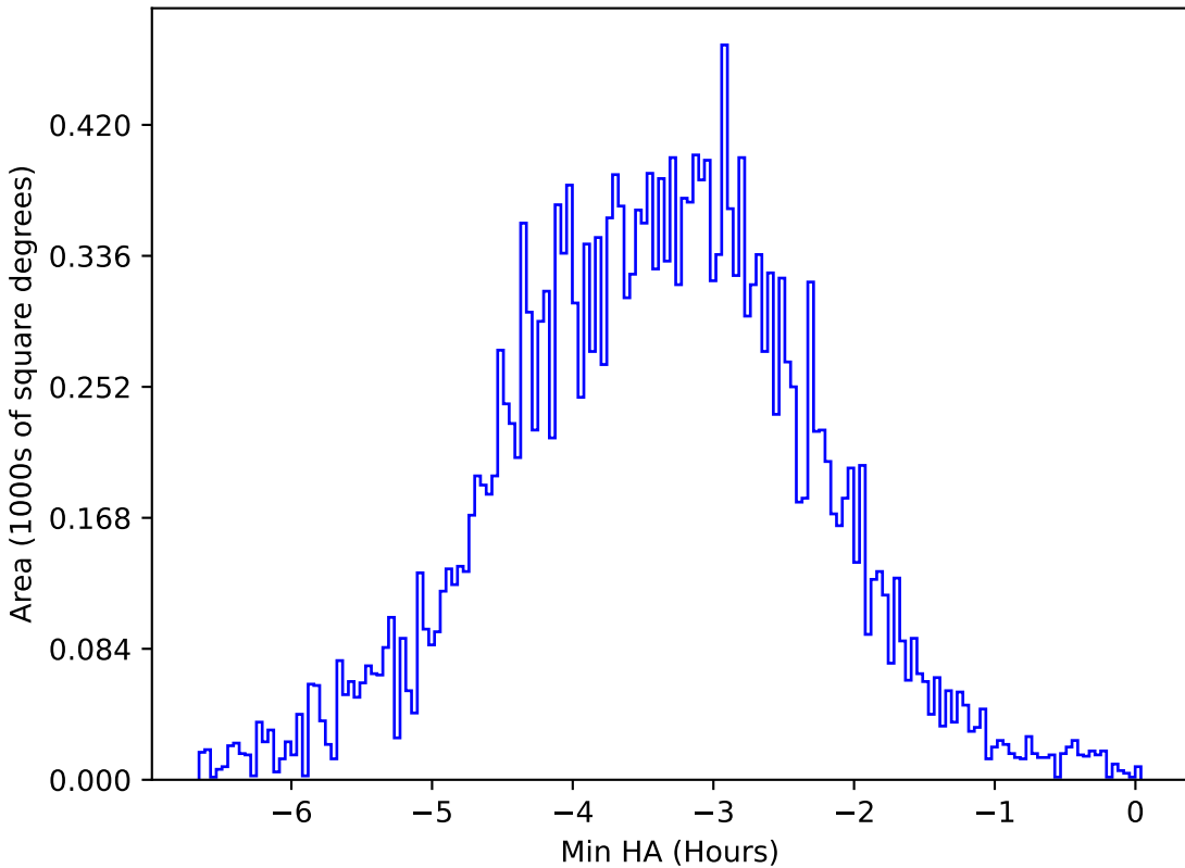
too_ignore_5_4v3.4_10yrs All sky y band: Min HA
