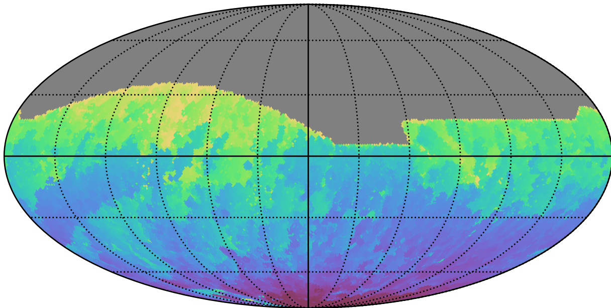
too_ignore_5_4v3.4_10yrs All sky i band: Min HA
