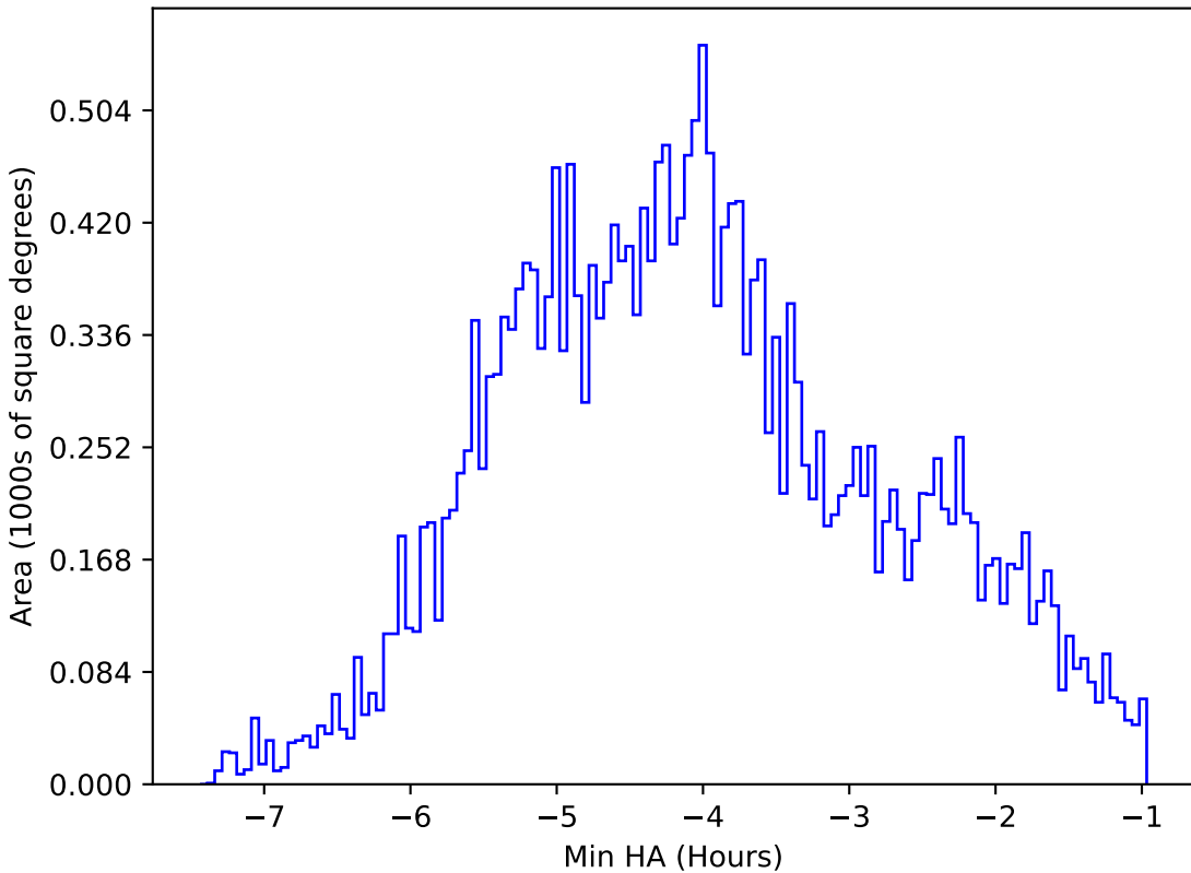
too_ignore_5_4v3.4_10yrs All sky i band: Min HA
