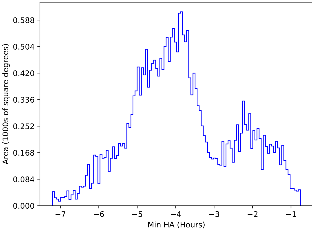
too_ignore_5_4v3.4_10yrs All sky g band: Min HA
