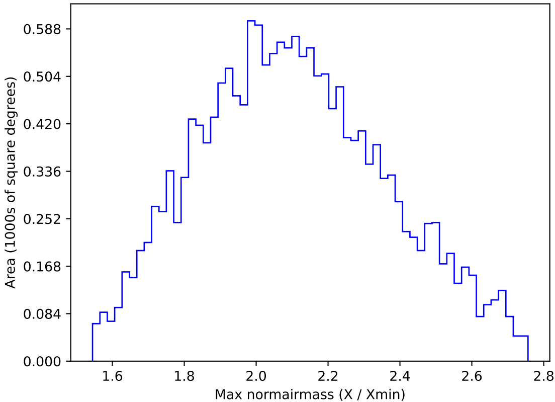
too_ignore_5_4v3.4_10yrs WFD y band: Max normairmass
