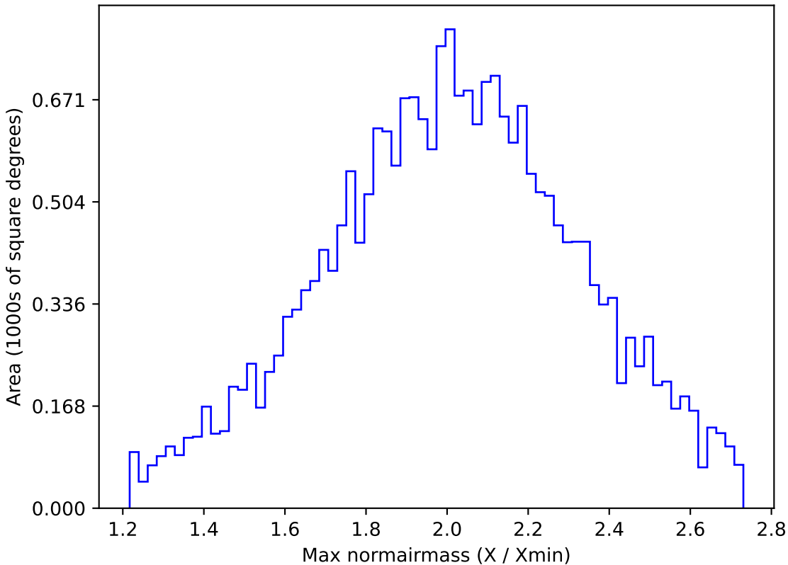
too_ignore_5_4v3.4_10yrs All sky y band: Max normairmass
