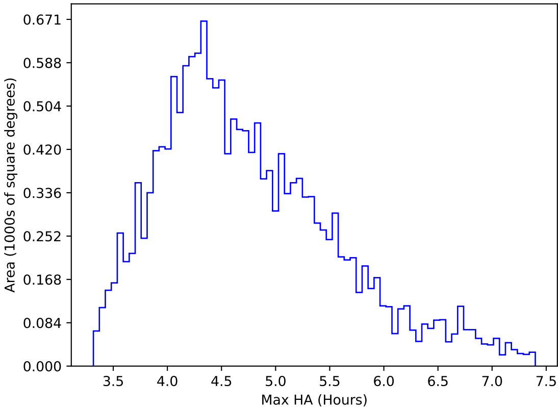
too_ignore_5_4v3.4_10yrs WFD y band: Max HA
